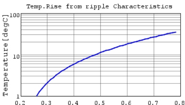
■ GJM1555C1H1R1BB01 Temp.rise 3GHz
